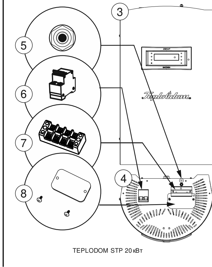
Рисунок 1. Общий вид стабилизатора и его функциональных элементов
