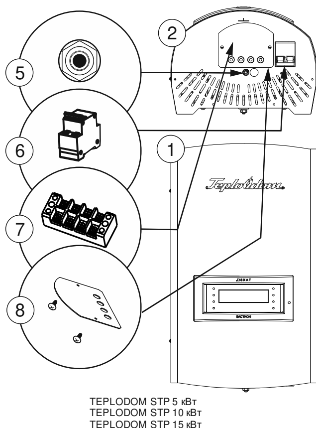
Рисунок 1. Общий вид стабилизатора и его функциональных элементов
